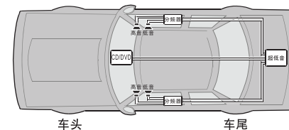
BC10.3-V安装布线图
