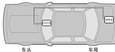
BC10.1-V安装布线图
